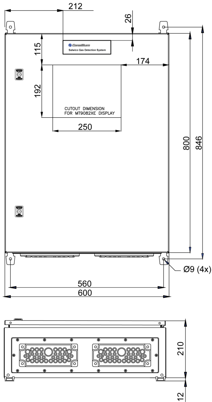
Afbeelding 1. Afmetingen kast
