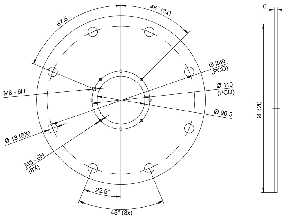
Afbeelding 2. Flensafmetingen PG11 &amp; PGE11 DIN200
