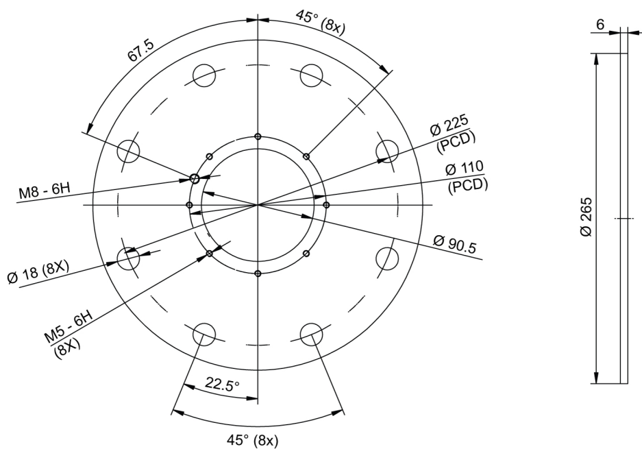
Afbeelding 1. Flensafmetingen PG11 & PGE11 DIN150
