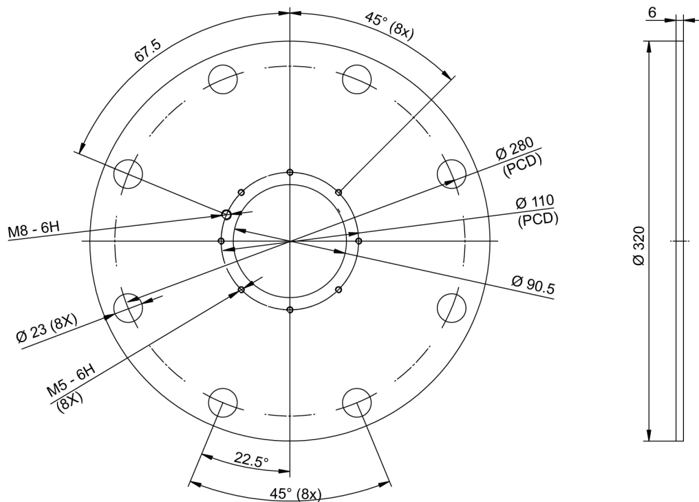
Afbeelding 4. Flensafmetingen PG11 &amp; PGE11 JIS200
